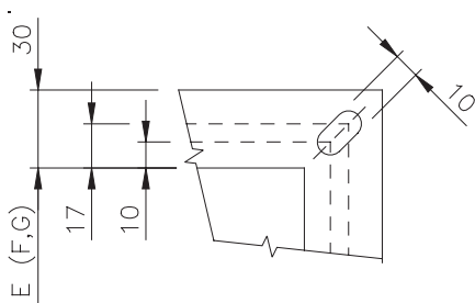
Flansch Abb. 5
