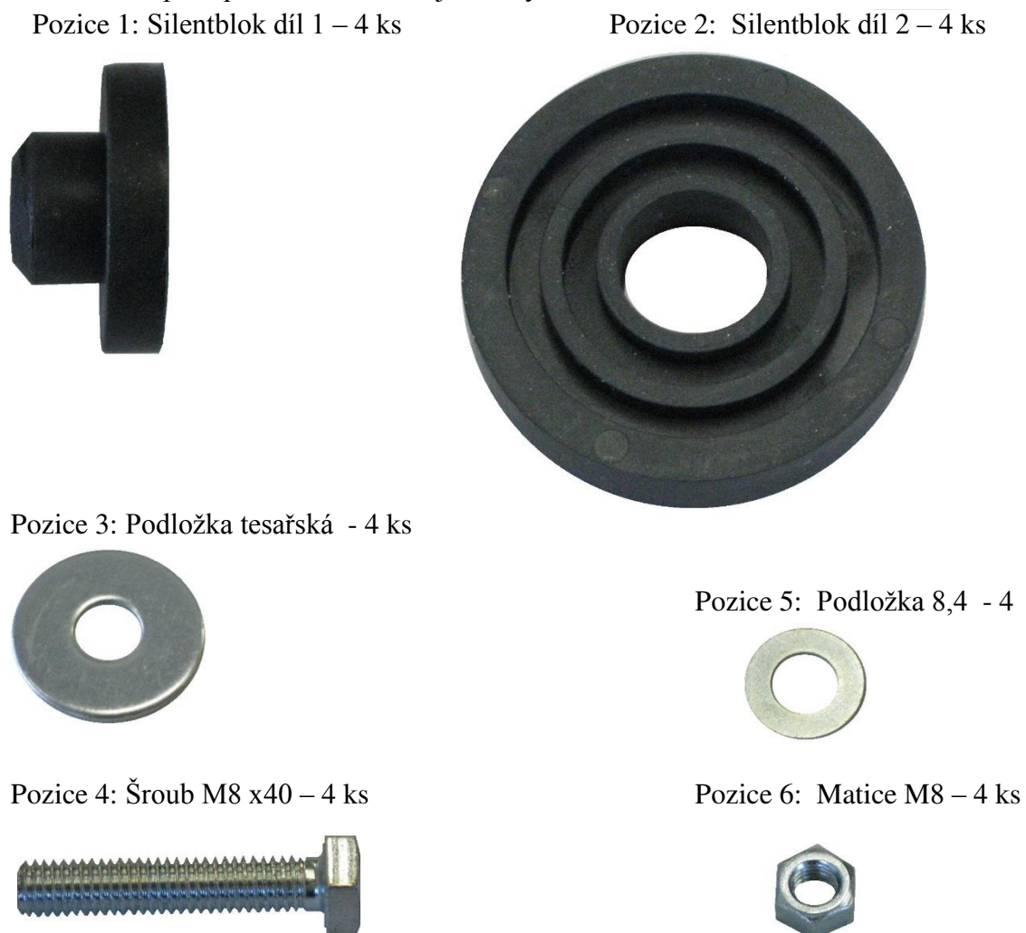
Obr. 3: Sada pro upevnění venkovní jednotky:
