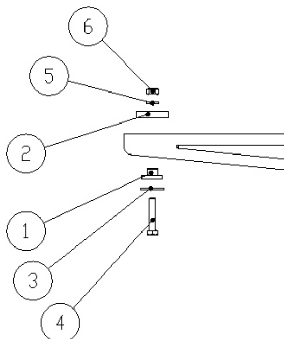
Obr. 5: Sestavení silentbloku pro připevnění venkovní jednotky
