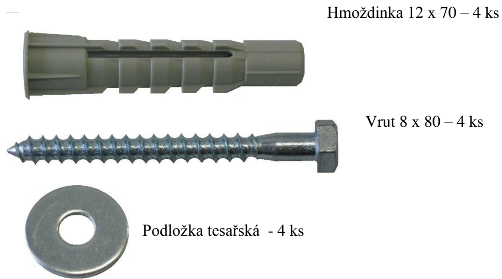
Obr. 2: Kotevní sada pro kotvení konzolí do zdi:
