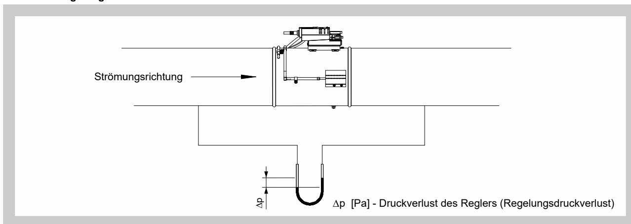
Abb. 3 Regelungsdruckverlust
