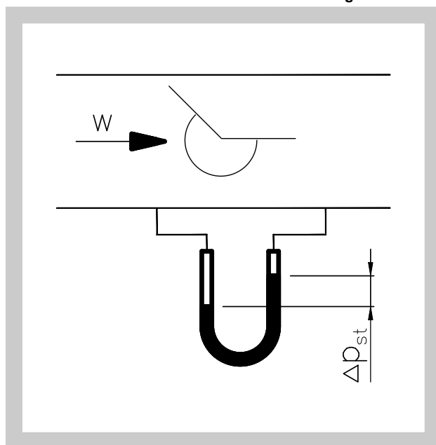
Abb. 10 Druckdifferenz am Volumenstromregler
