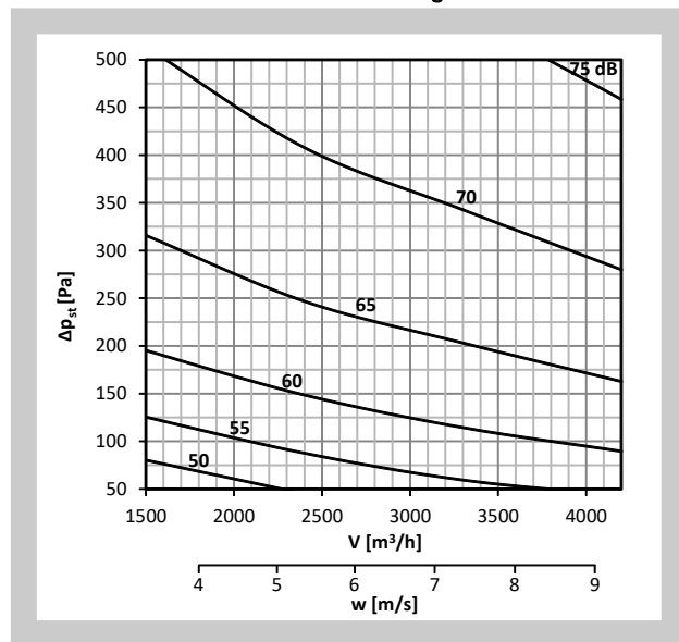
Diagramm Nr. 16 Schalleistungspegel L_{WA} [dB(A)] innerhalb der Anschlussleitung - 500x400
