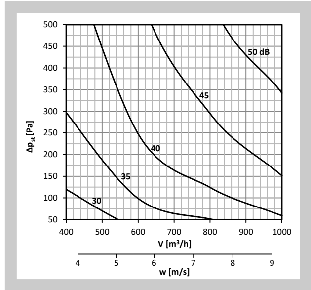
Diagramm Nr. 50 Schalleistungspegel L_{WA} [dB(A)] außerhalb der Anschlussleitung 300x100, isoliert
