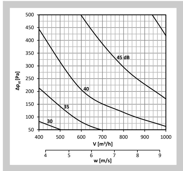
Diagramm Nr. 52 Schalleistungspegel L_{WA} [dB(A)] außerhalb der Anschlussleitung 300x200, isoliert
