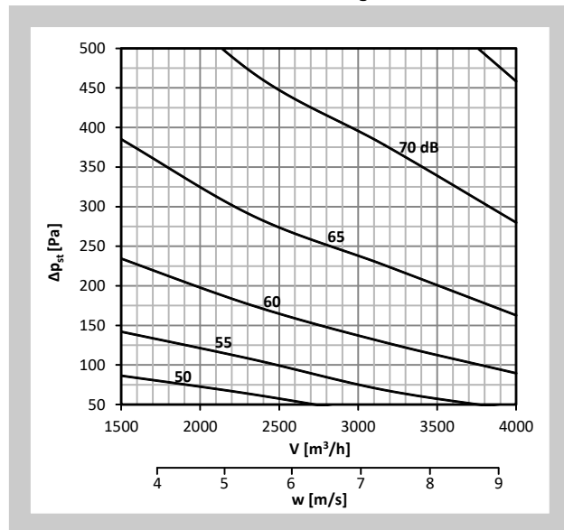
Diagramm Nr. 18 Schalleistungspegel L_{WA} [dB(A)] innerhalb der Anschlussleitung - 600x200
