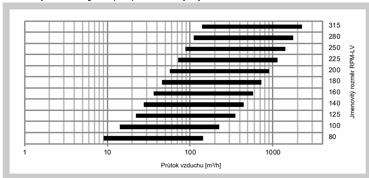
Obr. 16 Výběr velikosti regulátoru podle průtoku vzduchu [m³/h]
