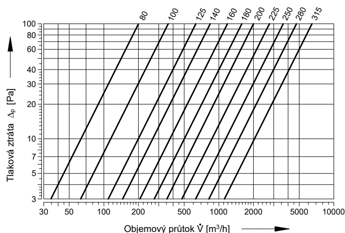
Diagram 8.1.1. Tlakové ztráty regulátoru (hodnoty platí při úplném otevření klapky regulátoru)
