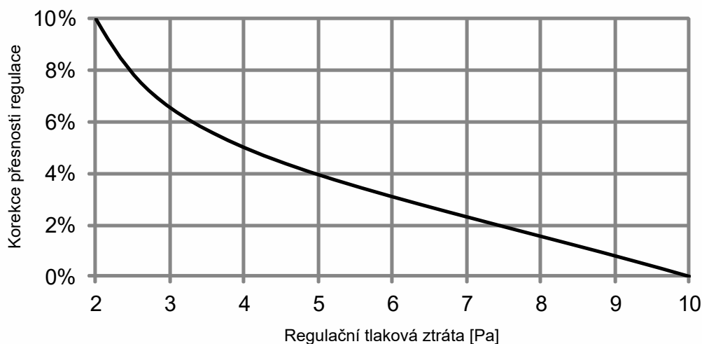
Graf 2 Korekce přesnosti regulace pro velmi nízké regulační tlakové ztráty
