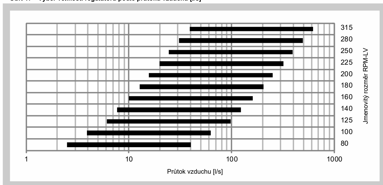
Obr. 17 Výběr velikosti regulátoru podle průtoku vzduchu [l/s]
