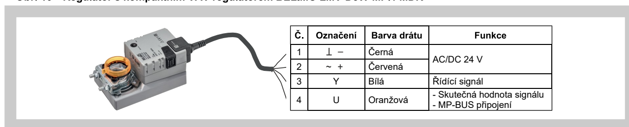
Obr. 11 Regulace průtoku vzduchu pomocí pohonu LMV-D3W-MP.1 MDK
