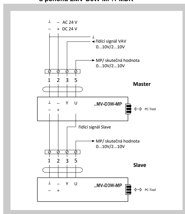
Obr. 12 Regulace průtoku v zapojení MASTER-SLAVE u pohonů LMV-D3W-MP.1 MDK
