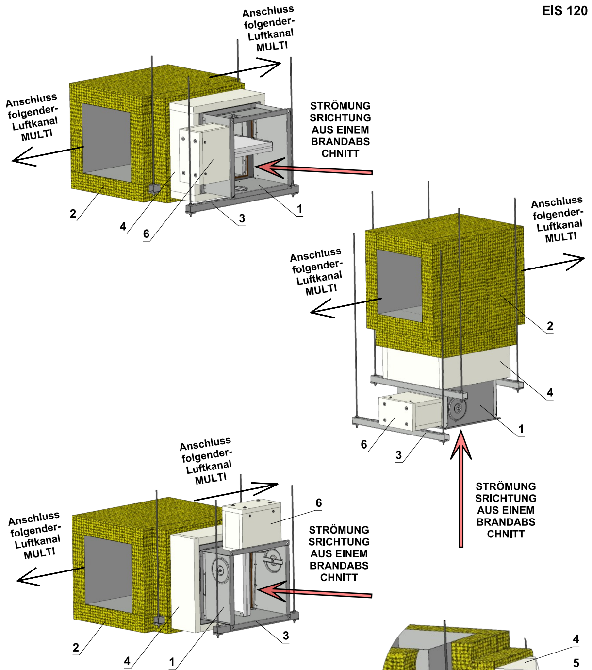
Abb. 48 Installation in einen horizontalen Luftkanal MULTI / MULTI - Isolierung mit Steinwolle
