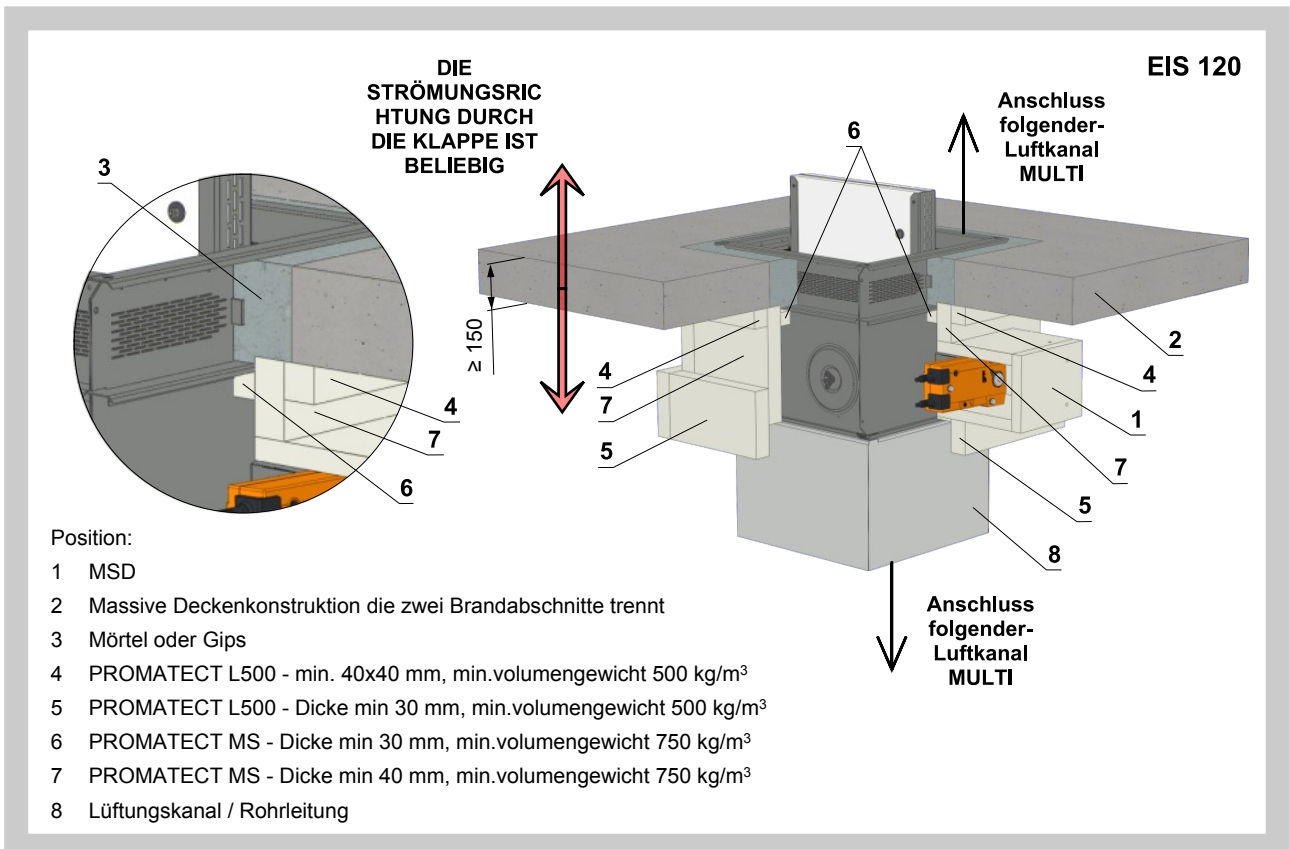
Abb. 43 Trennkonstruktion zwischen Luftkanal MULTI / MULTI - Isolierung mit Kalk-Zement-Boards - Mörtel oder Gips - Die Montage der Klappe ist von der Ober- sowie von der Unterseite der Deckenkonstruktion möglich.
