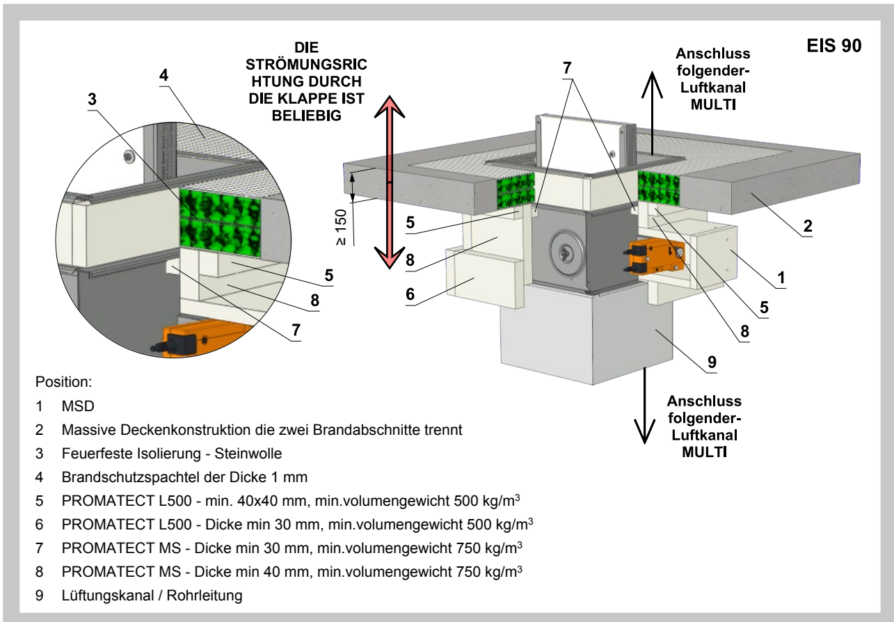
Abb. 45 Trennkonstruktion zwischen Luftkanal MULTI / MULTI - Isolierung mit Kalk-Zement-Boards - Weichschott - Die Montage der Klappe ist von der Ober- sowie von der Unterseite der Deckenkonstruktion möglich.
