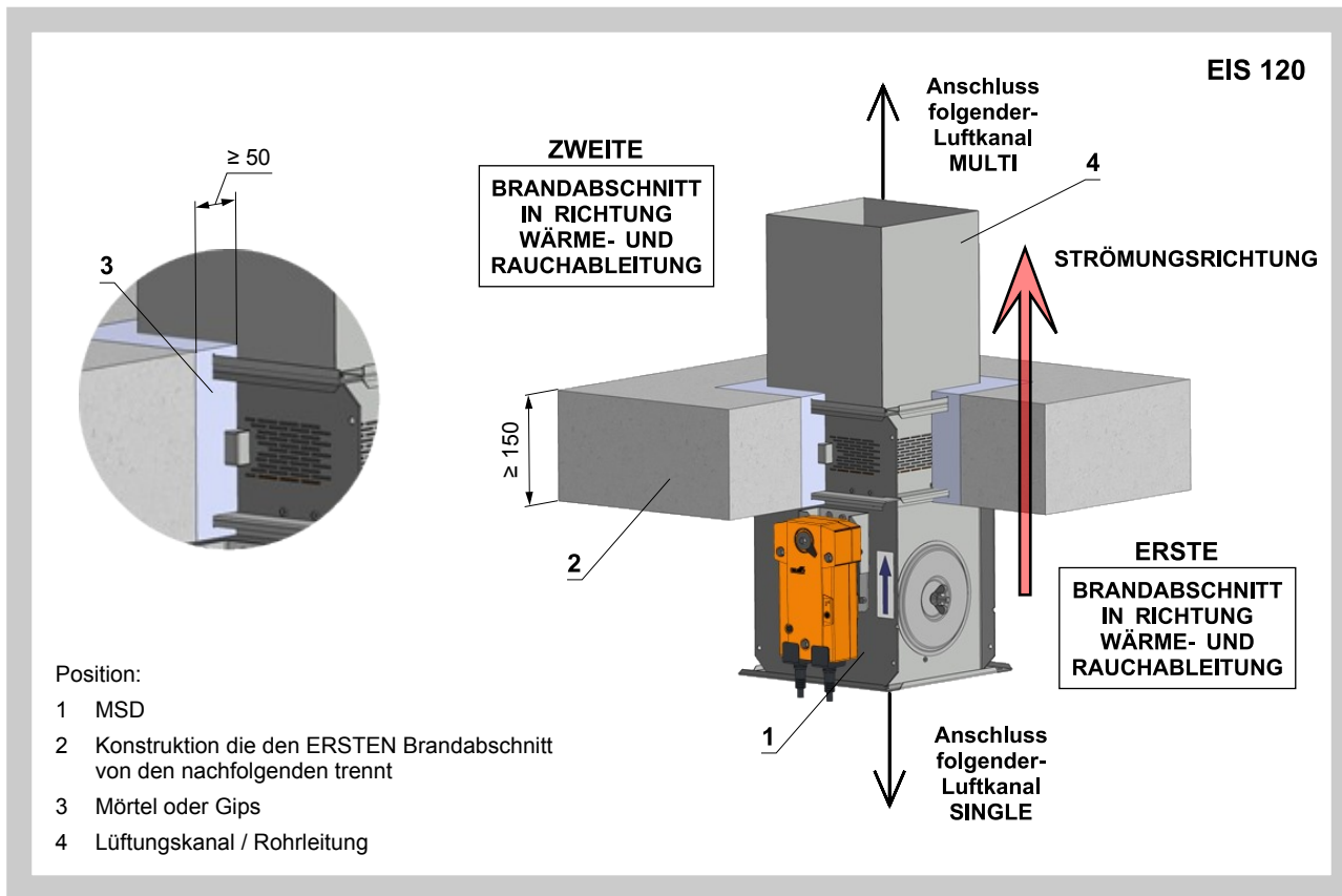
Abb. 40 Trennkonstruktion zwischen Luftkanal SINGLE / MULTI - Mörtel oder Gips
