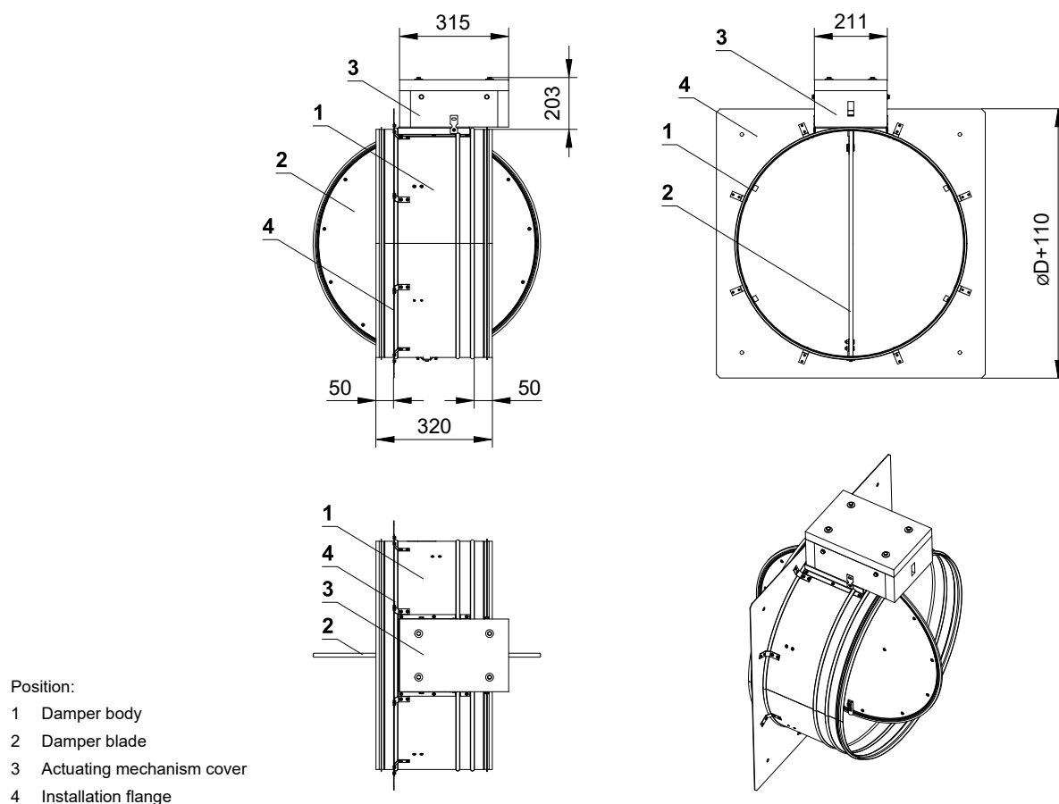
Fig. 6 Damper SEDS-R
