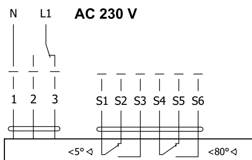
Fig. 11 Actuator BELIMO BEE 230
