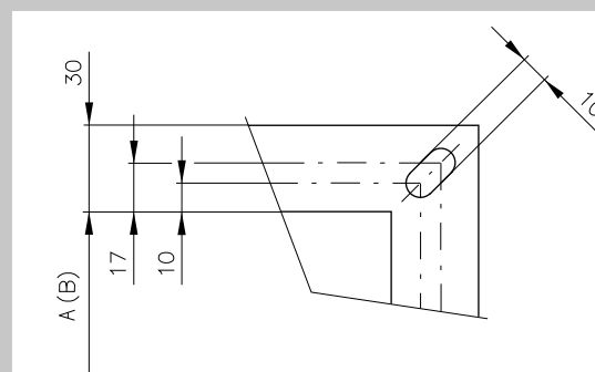
Fig. 5 Flanges
