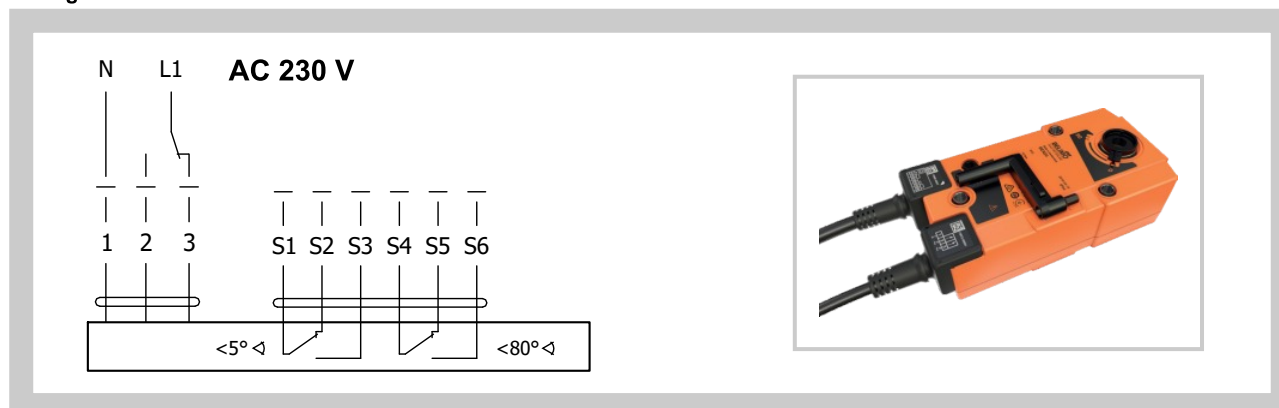
Fig. 9 Actuator BELIMO BEN 230
