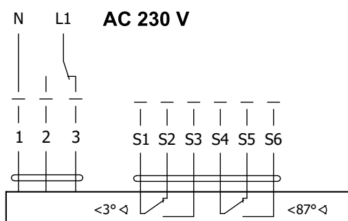
Fig. 13 Actuator BELIMO BE 230-12
