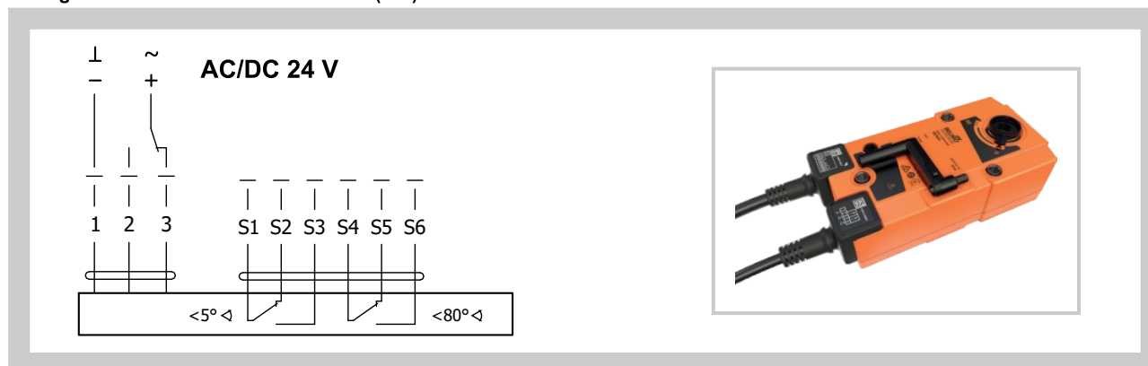
Fig. 8 Actuator BELIMO BEN 24(-ST)
