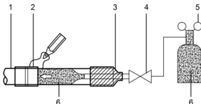
Obr. 17: Pájení v dusíku
