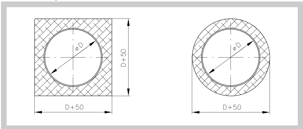
Abb. 8 Bauöffnung
