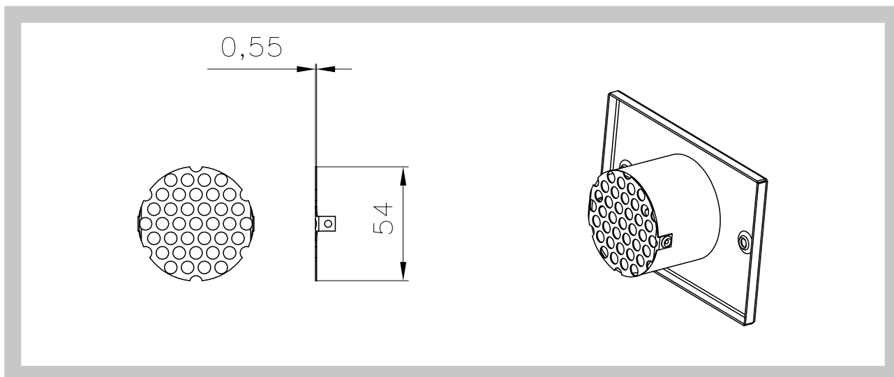
Abb. 3 Lochblecheinsatz
