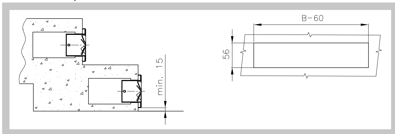
Abb. 4 Einbaubeispiel
