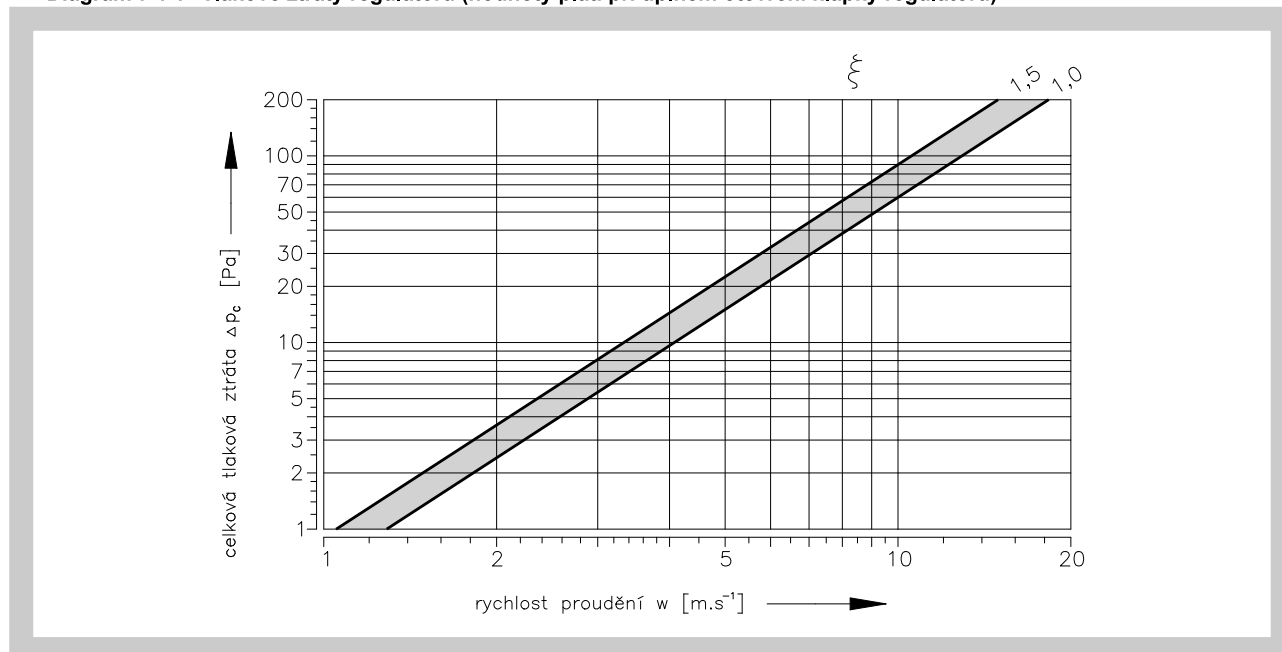
Diagram 7.1.1. Tlakové ztráty regulátoru (hodnoty platí při úplném otevření klapky regulátoru)
