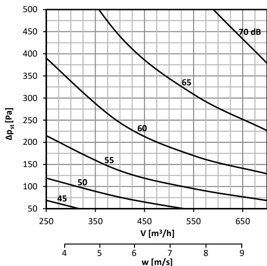
Graf č. 3 Hladina akustického výkonu L_{WA} [dB(A)] vyzářeného do potrubí 200x200
