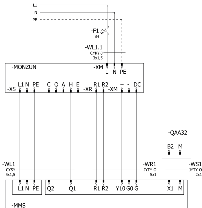
Obr. 2: Schéma propojení ohříváče MONZUN s ovládací skříňkou MMS
